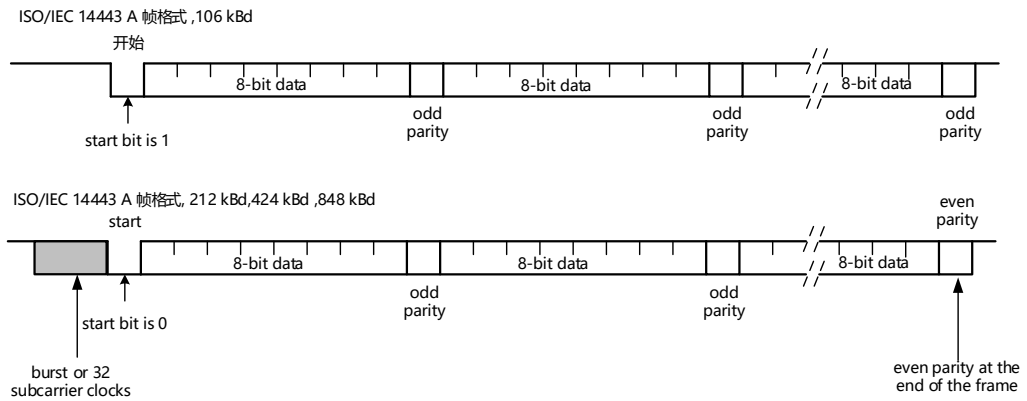
图 6.3 ISO/IEC 14443A 协议数据编码与帧结构
