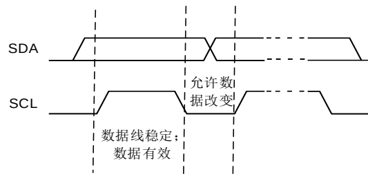
图 8.6 I²C 总线比特传输
