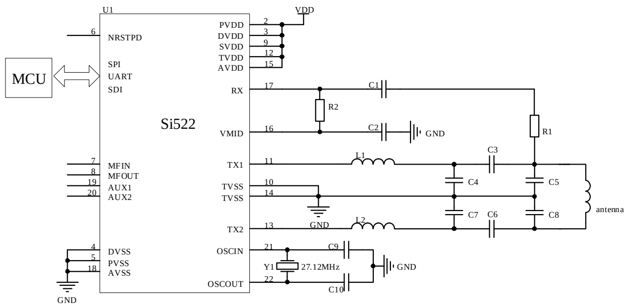
图 10-1 典型应用图-1
