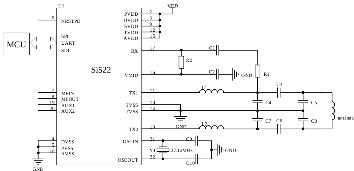
图 10-2 典型应用图-2
