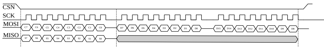
图 7-4 SPI 写操作
