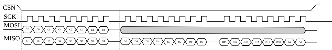
图 7-3 SPI 读操作
