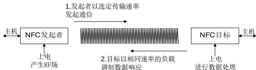
图 6.8 被动通信模式
