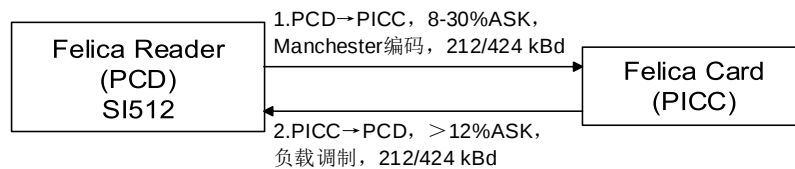
图 6.4 Felica 读卡器模式通信示意图
