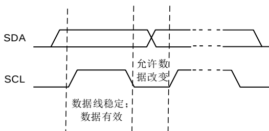
图 8.6 I 2 C 总线比特传输
