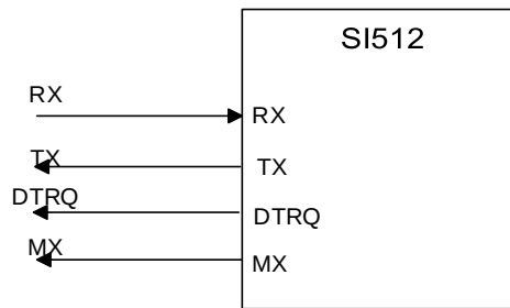
图 8.2 UART 接口
