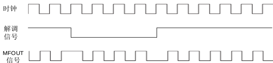
图 10.5 SAM 模式 MFOUT 信号波形示意图
