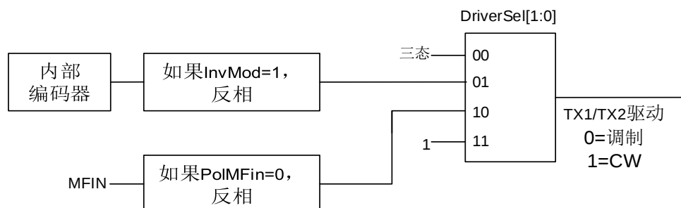
图 10.2 TX1 和 TX2 串行数据转换
