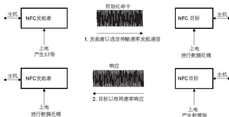
图 6.7 主动通信模式
