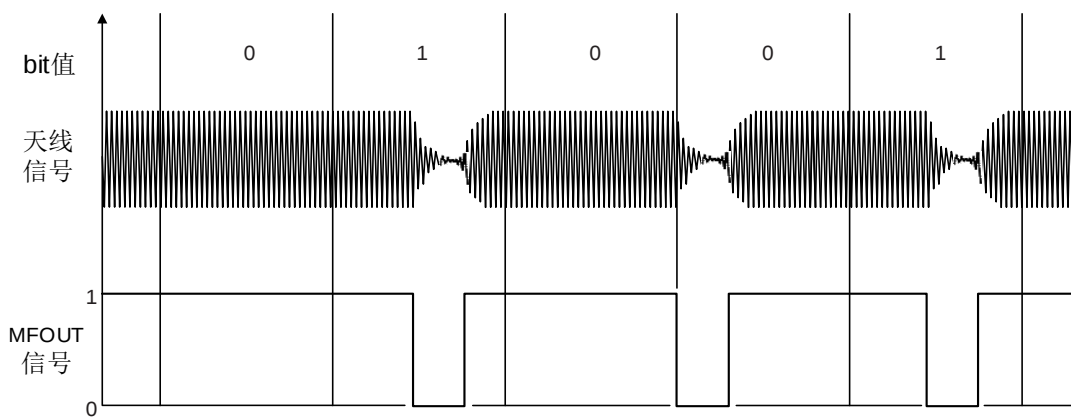
图 10.6 MIFARE 卡 SAM 模式 MFOUT 信号波形示意图
