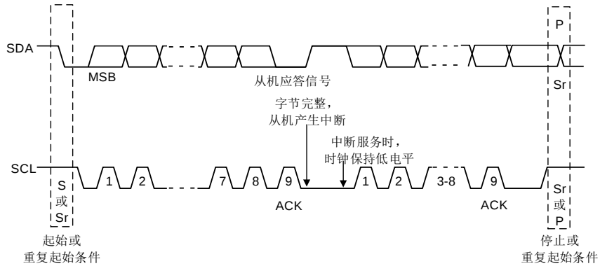
图 8.9 I2C 总线数据传输示意图
