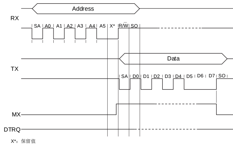
图 8.3 UART 读数据时序图
