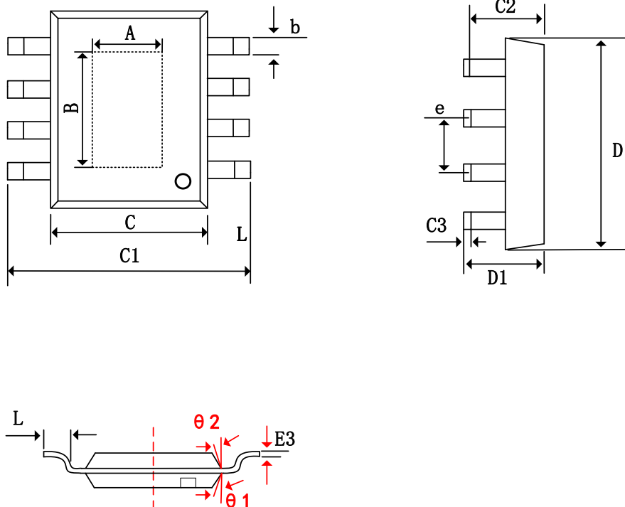
ESOP-8
