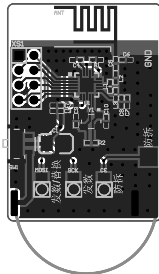
图 9-2 片上天线布线图 (0402 元件)
