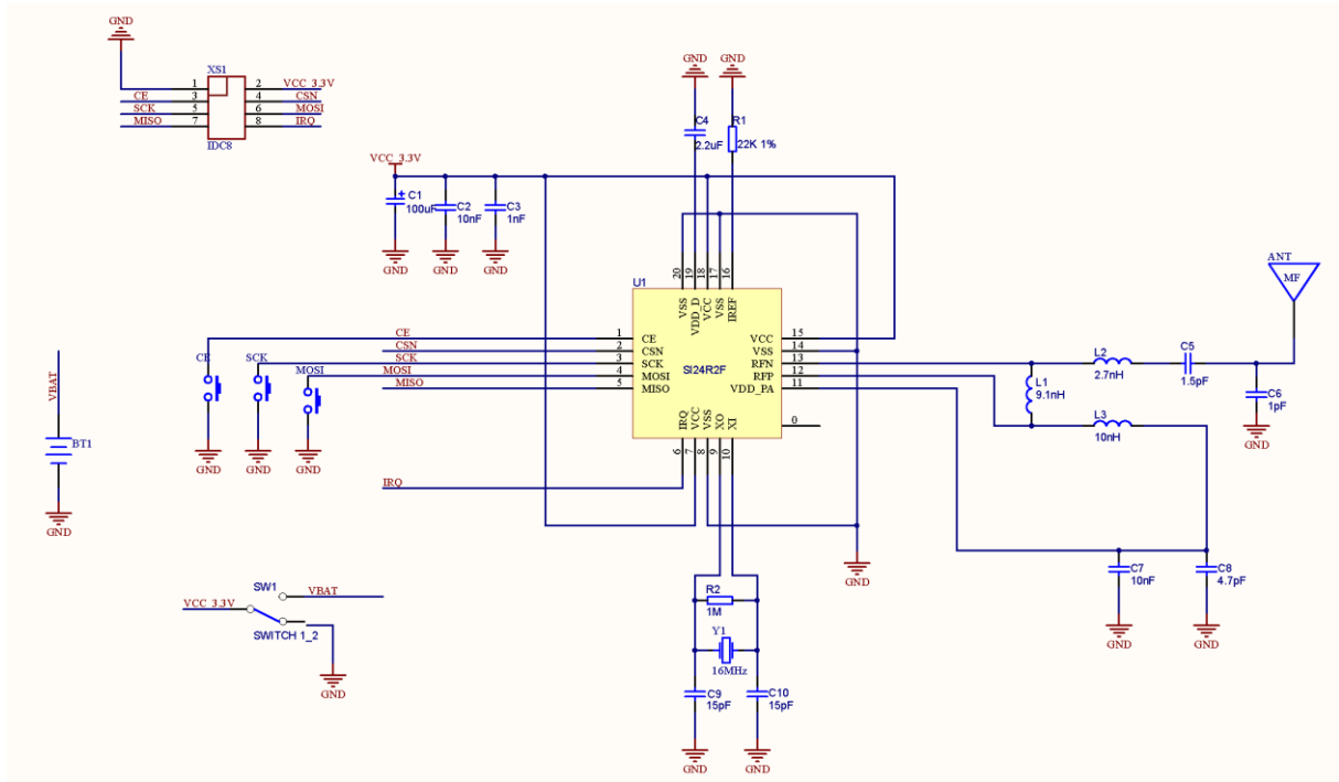
图 9-1 典型应用原理图
