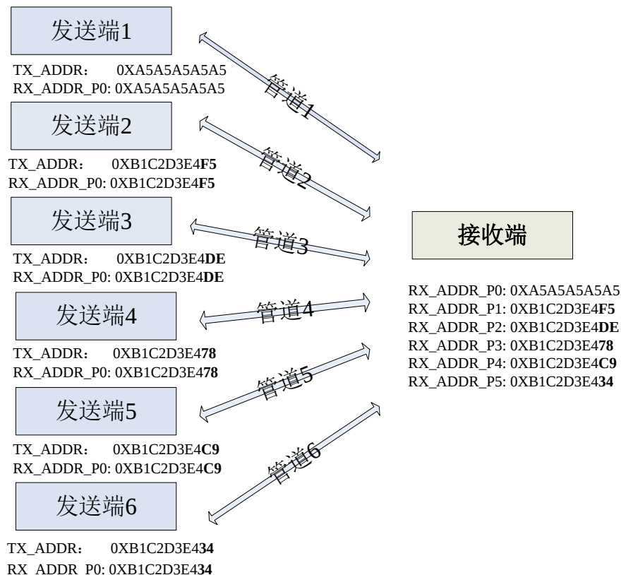
图 20-9 多管道通信模式
