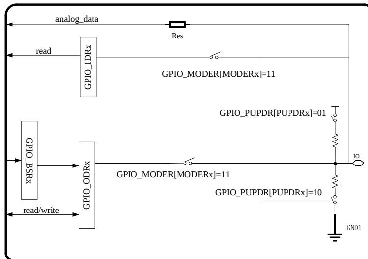
图 5-4 GPIO 模拟功能配置原理图
