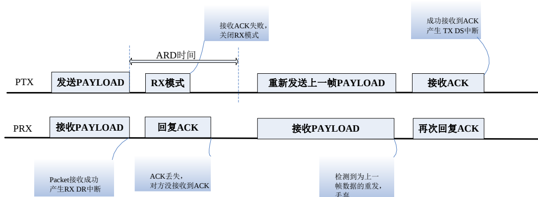
图 20-7 无 ACK PAYLOAD 通信模式
