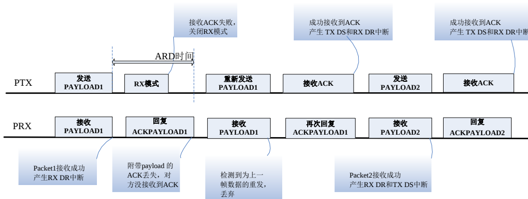
图 20-8 带 ACK PAYLOAD 通信模式
