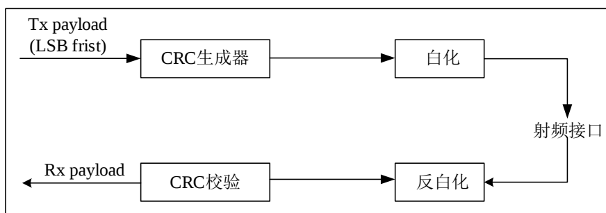
图 20-5 蓝牙数据包数据流
