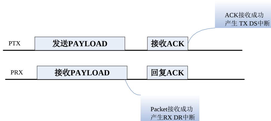
图 20-6 示为 ACK 模式下的一次通信完成。
