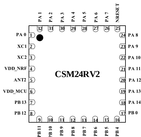
图 1-1 管脚信息图（5x5 mm QFN32）
