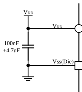
图 24-1 电源供电方案
