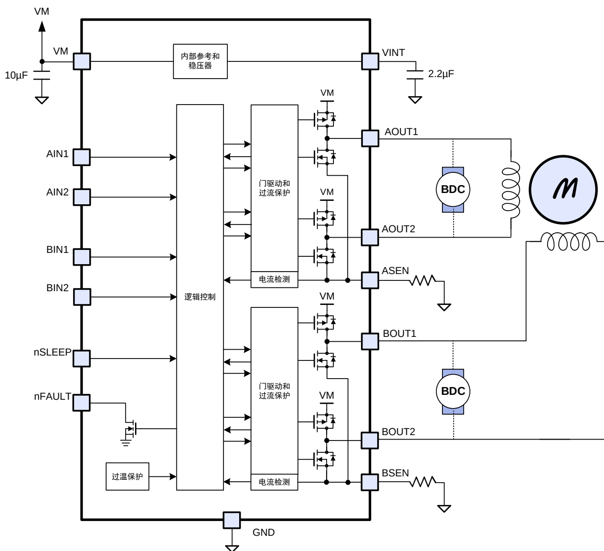
图3. LTK8833C功能框图
