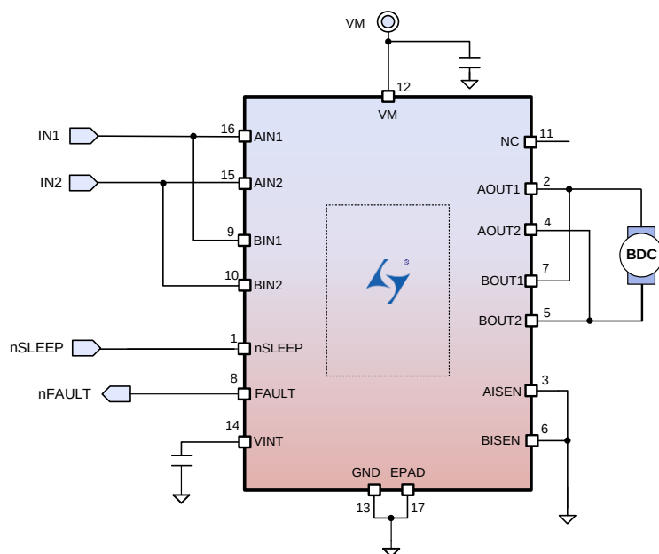
图7. 并联模式
