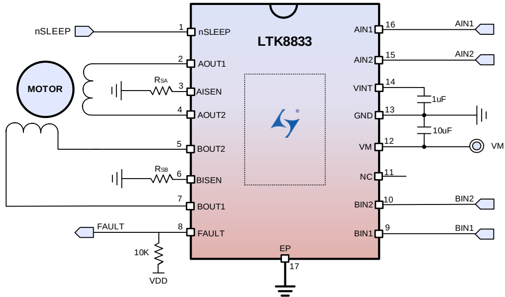
图8. 典型应用图
