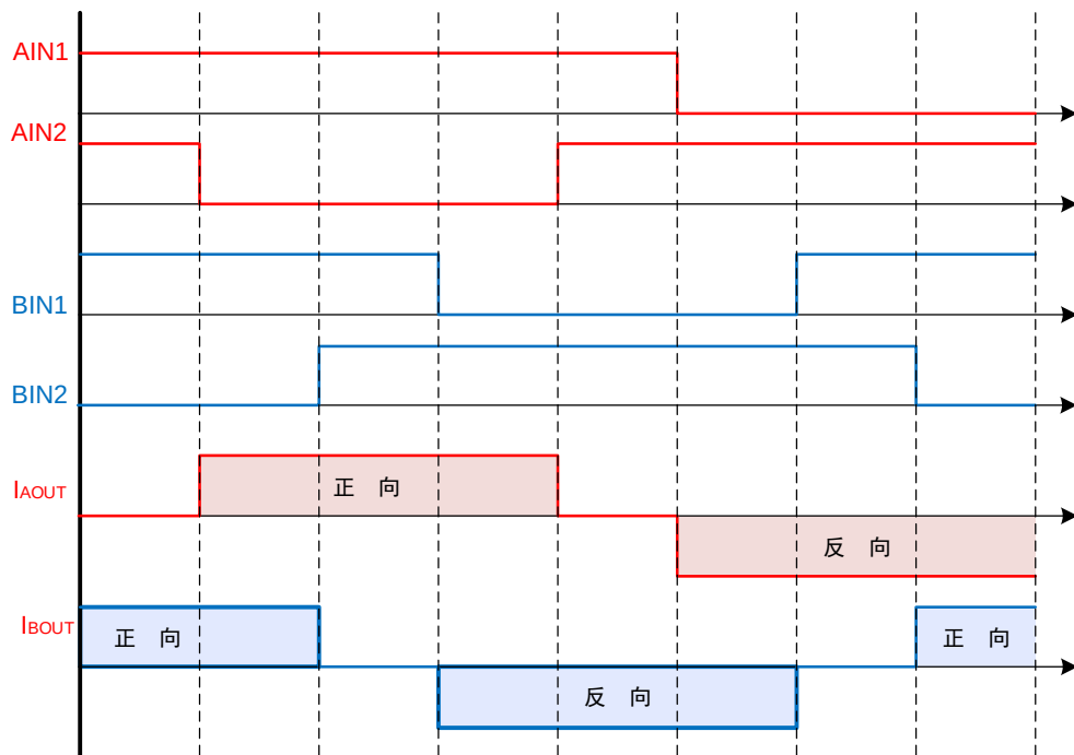
图 10. 半步进模式
