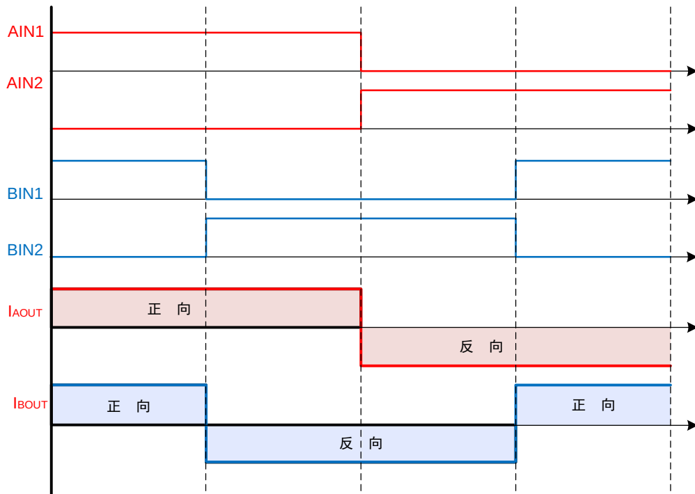
图9. 全步进模式
