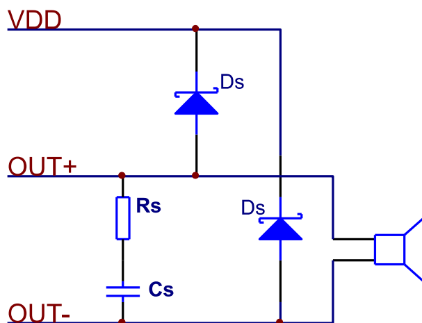
图6. 输出端的连接
