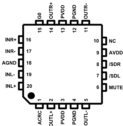
20引脚QFN 顶视图
