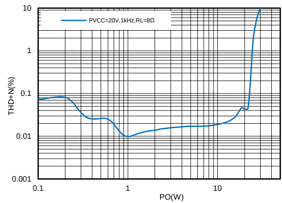
图36. 20V供电8Ω负载THD+N曲线PBTl
