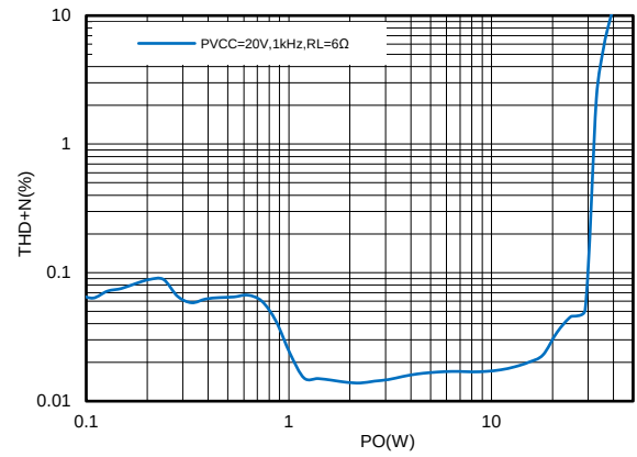
图32. 20V供电6Ω负载THD+N曲线PBTl
