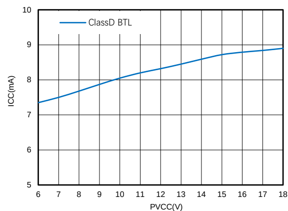
图23. 不同供电电压下的静态电流
