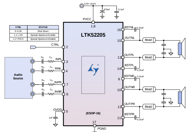
图1. LTK52205 简化应用原理图
