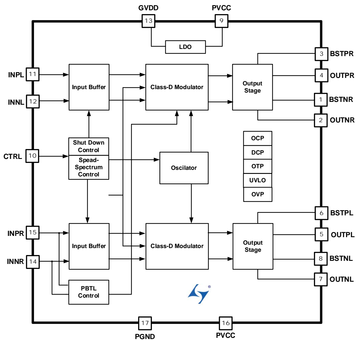
图 3. LTK52204 功能框图示意图
