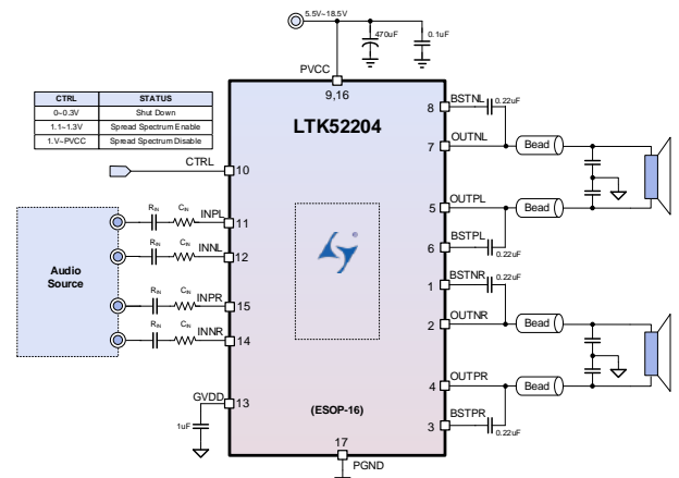
图1. LTK52204 简化应用原理图
