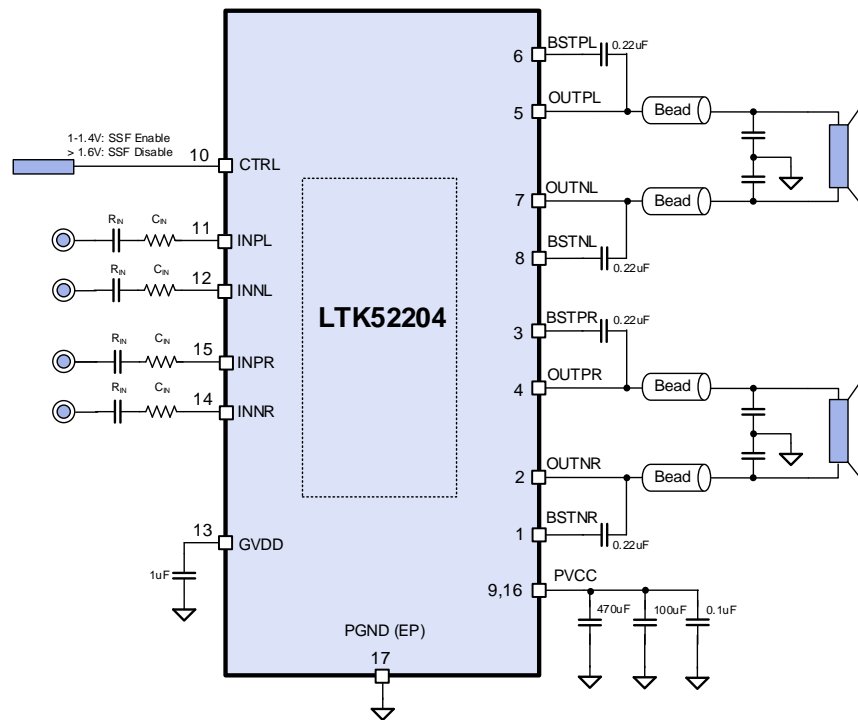
图 4. 差分输入立体声 BTL 输出模式
