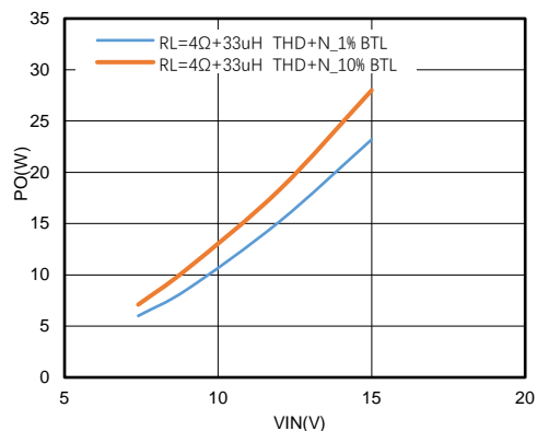
图8. 4Ω负载下不同电源电压的THD+N
