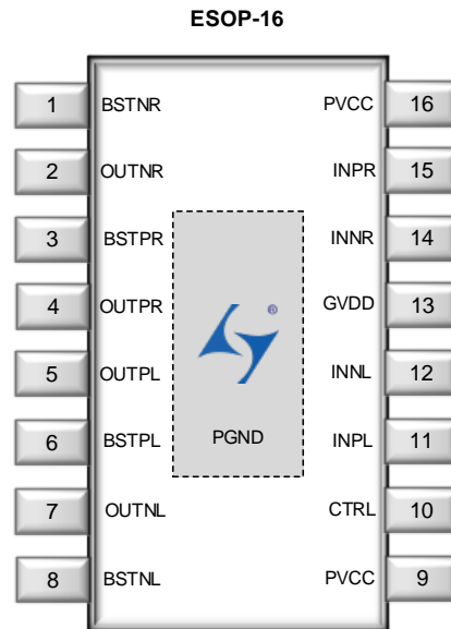
图2. LTK52204 管脚说明
