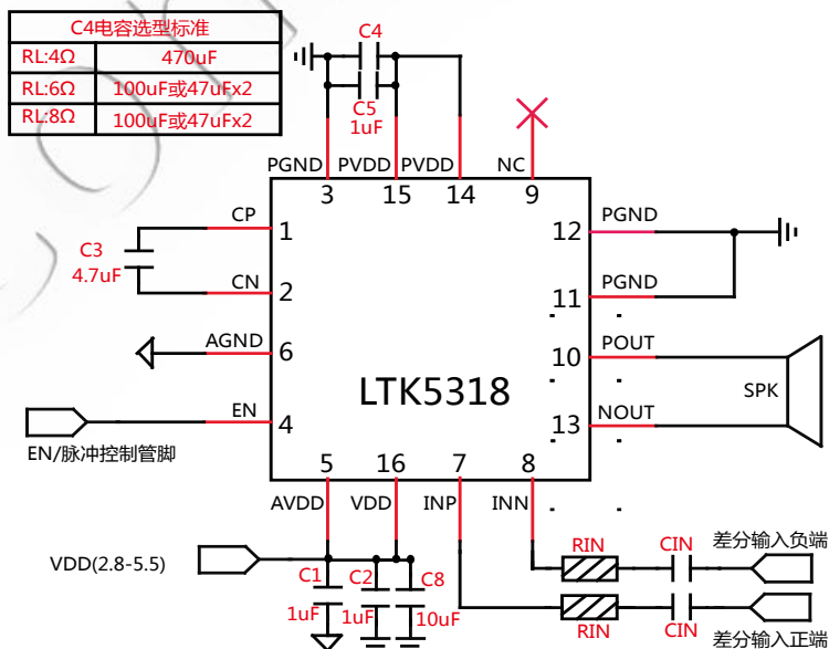
图 1 典型应用图
