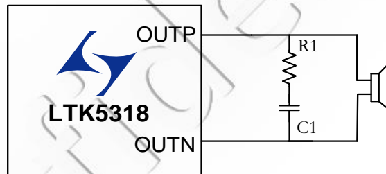
图 5 缓冲网络
