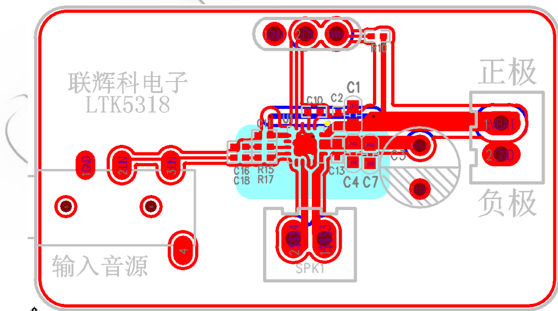
图 4 Demo 板设计图 (仅供参考)
